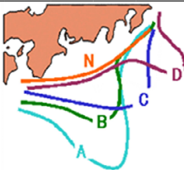
図1 黒潮流型
