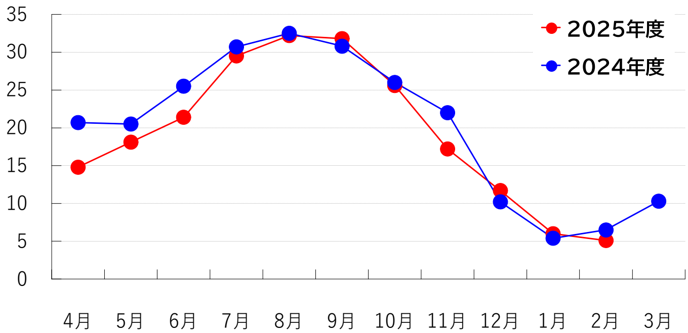
内浦 表層水温(℃)
