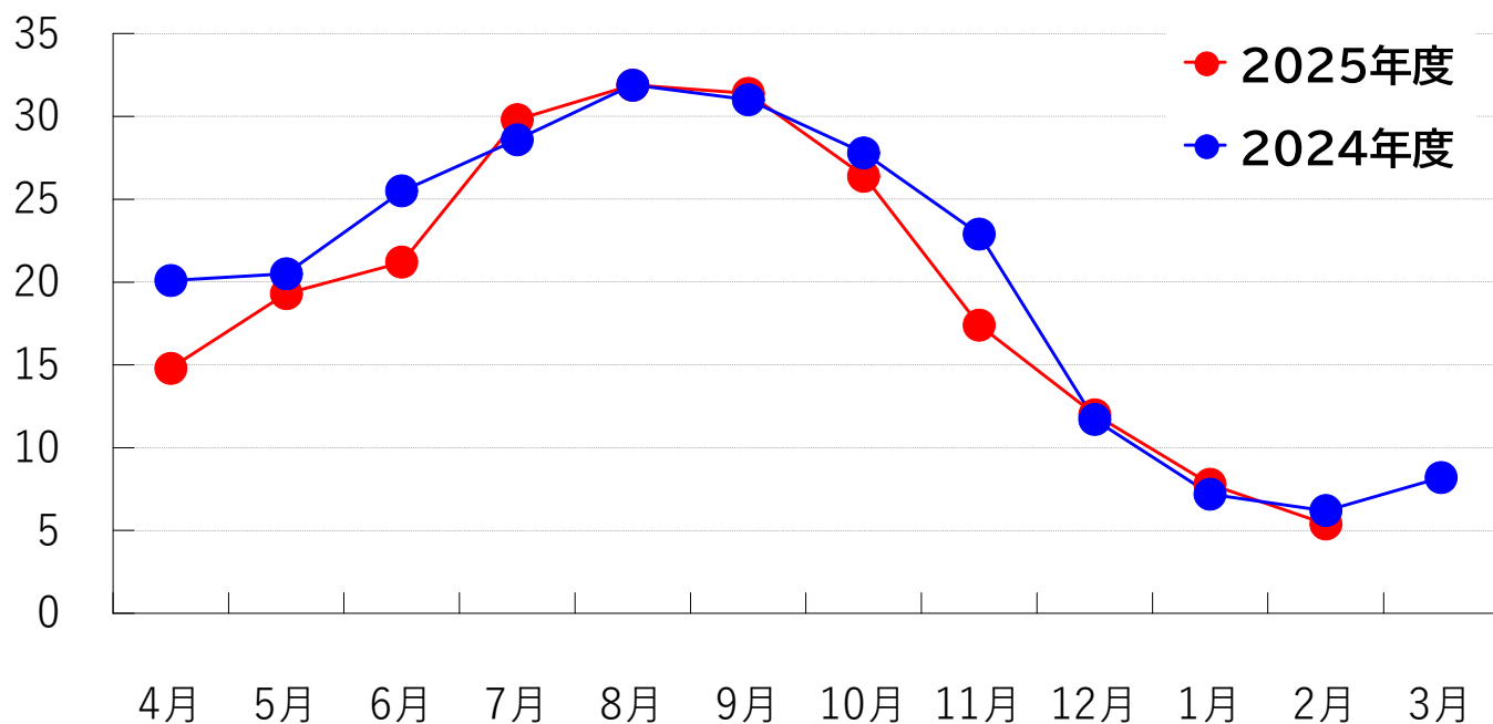
松見ヶ浦 表層水温(℃)
