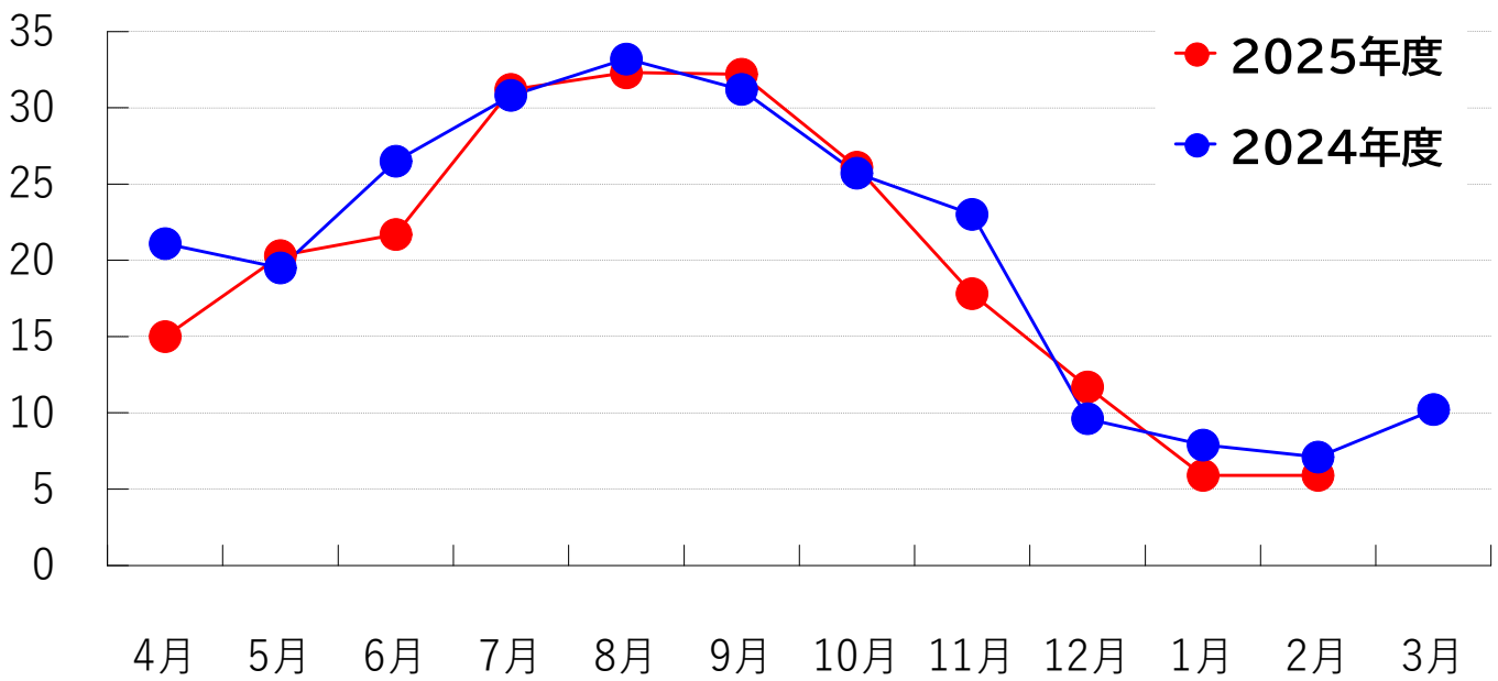
細江湖 表層水温(℃)
