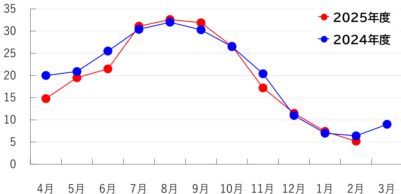
猪鼻湖 表層水温(℃)
