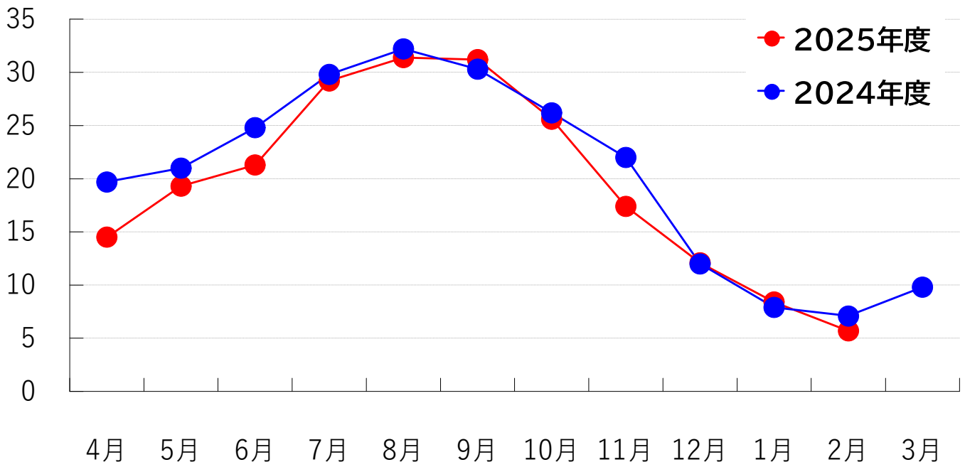
湖心 表層水温(℃)
