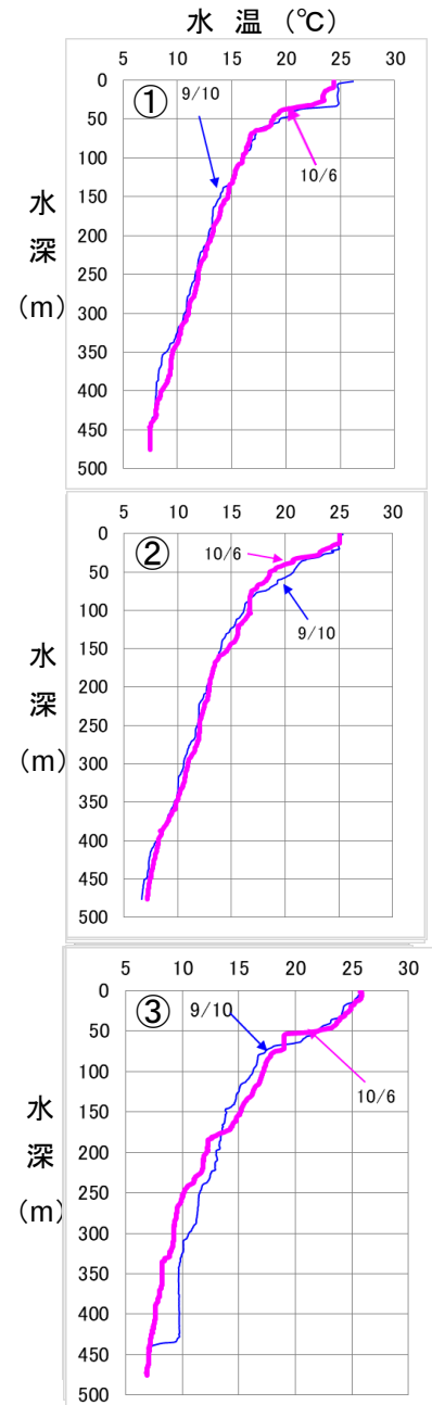
調査地点ごとの水温の鉛直図 (過去2回の調査結果)
