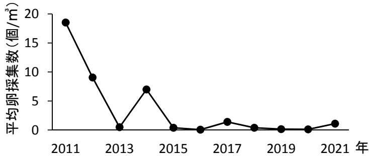
図2 カタクチイワシ卵の採集数の推移
