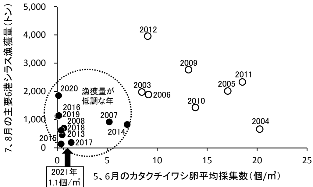
図3 5、6月カタクチイワシ卵平均採集数と7、8月主要6港シラス水揚量の関係（図中の数字は西暦年）
