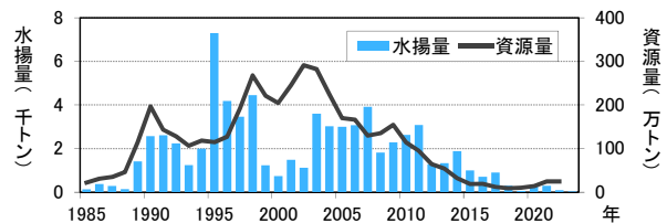
図 2 県内カタクチイワシ水揚量と カタクチイワシ太平洋系群の資源量の推移
