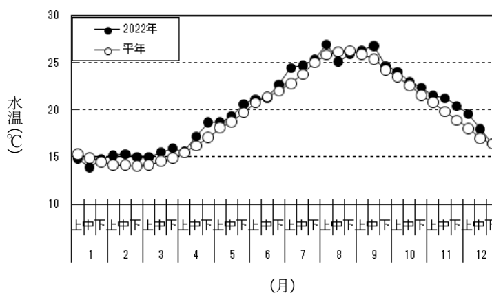
図 2 焼津の定地水温
