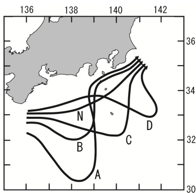
図 1 黒潮流路の型
