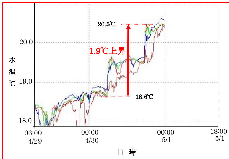
図1 2022年4月30日06時～5月1日00時までの妻良水温の変化
