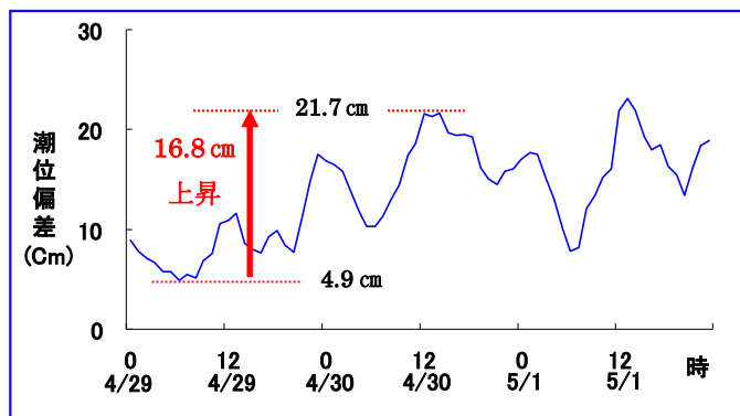
図2 石廊崎の潮位偏差の変化
