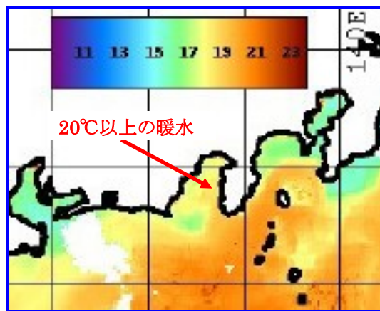
図3 2022年4月30日の気象衛星ひまわり画像 (三重県水産研究所HPより)
