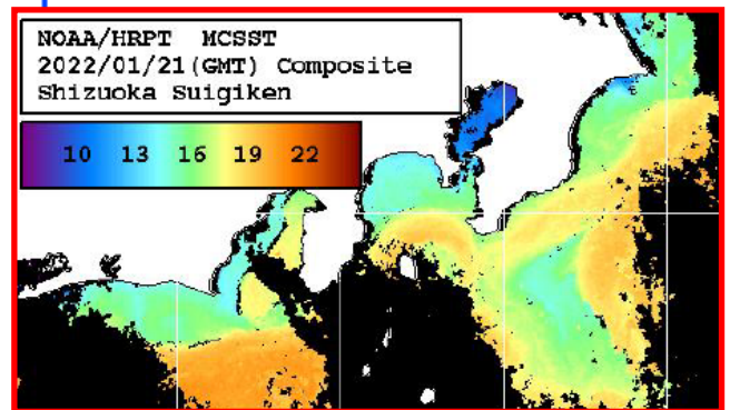
図2 NOAA水温画像(静岡水技研HPから) (1月21日)
