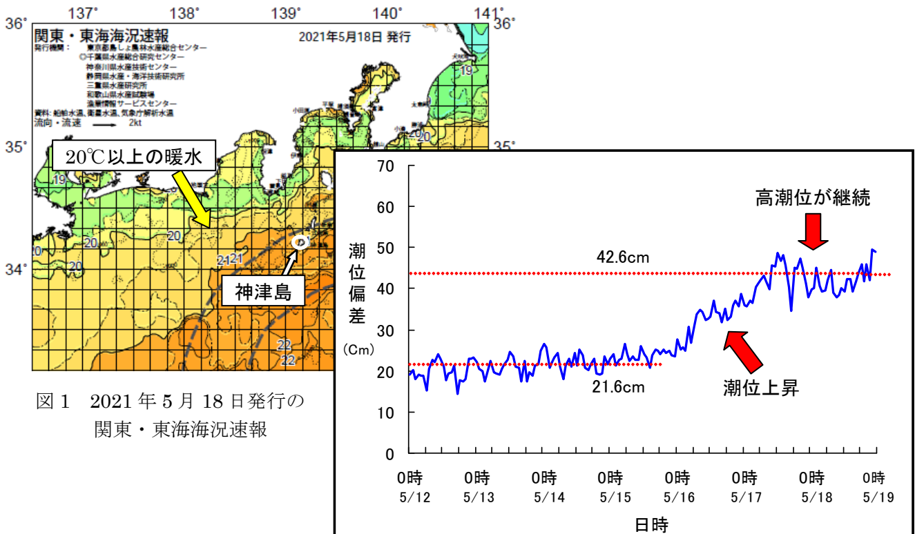
図2 2021年5月12日から5月18日までの神津島の潮位偏差
