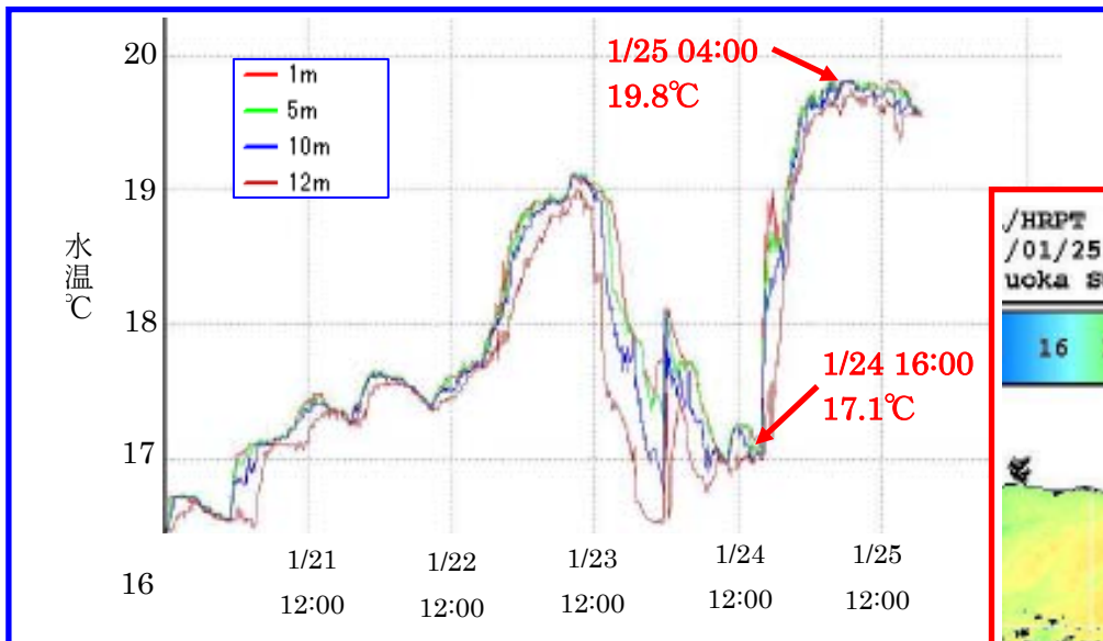
図1 妻良水温観測ブイの水温
