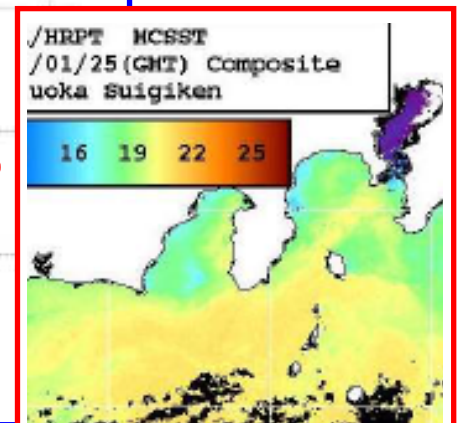
図2 1月25日の人工衛星ノアの画像
