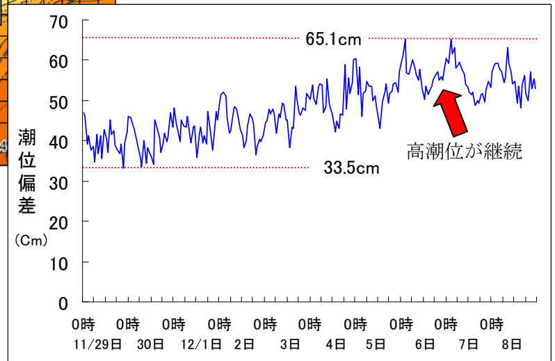
図2 2020年11月29日から12月8日までの 神津島の潮位偏差
