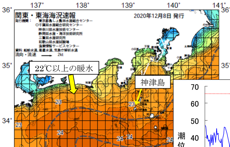
図1 2020年12月8日発行の 関東・東海海況速報
