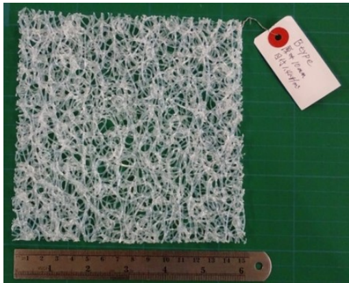
図7 樹脂繊維製移植基盤
