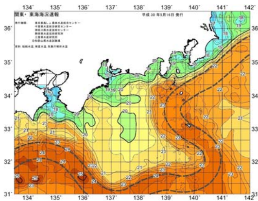
図 1 関東・東海海況速報(5 月 16 日)
