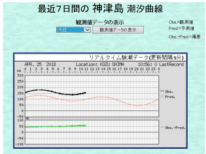
第2図 4月25日の神津島の潮汐曲線
