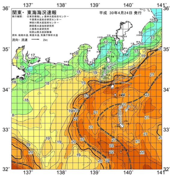
第1図 4月24日の関東・東海海況速報
