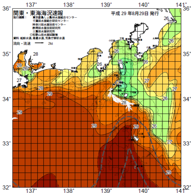
第1図 8月29日発行の関東・東海海況速報
